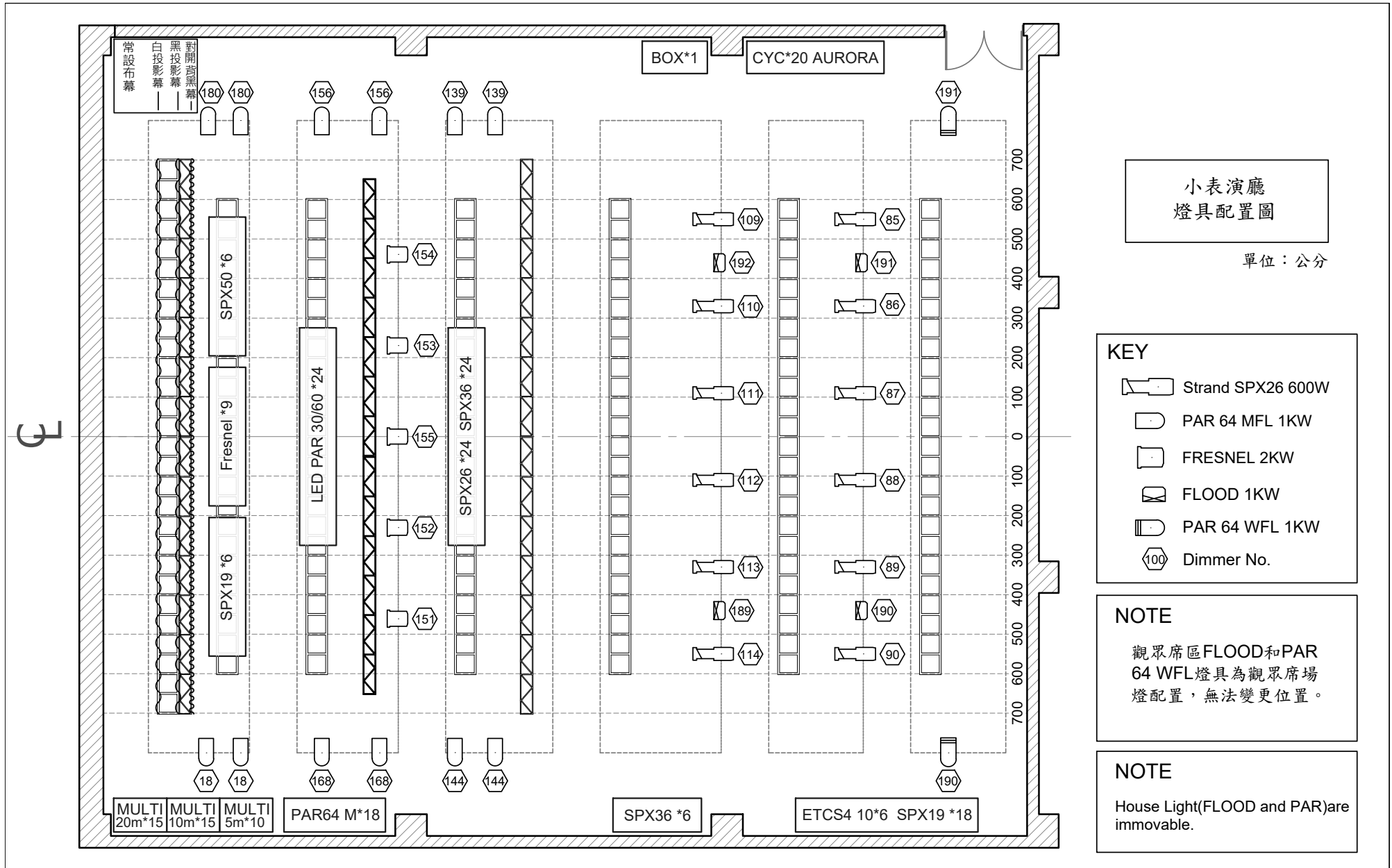
圖 (六) 小表演廳_燈具配置圖 (單位：公分) Figure(6) Experimental Theatre _Light Plot (Unit: cm)
