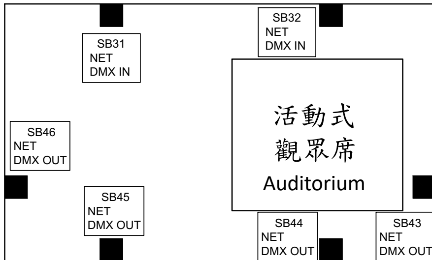
圖 (七) 小表演廳_燈光訊號盒位置圖 Figure(7) Experimental Theatre_Lighting Signal Chart
