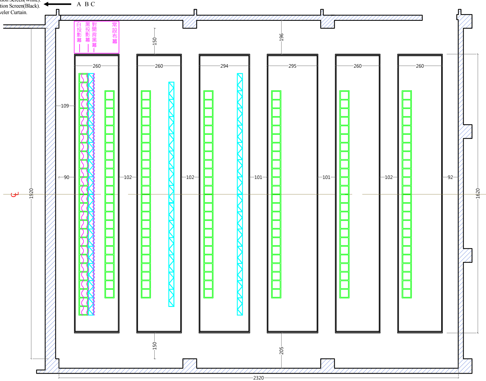
圖 (四) 小表演廳_3F空間平面圖 (單位: 公分) Figure(4) Experimental Theatre_3rd Floor Plan (Unit: cm)
