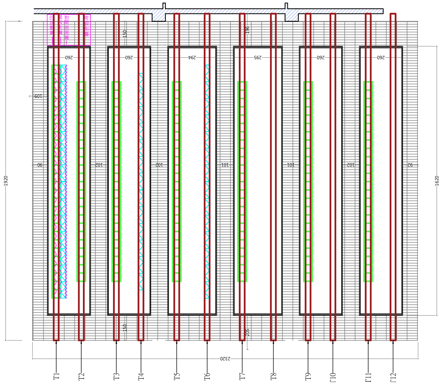
圖 (五) 小表演廳_馬達軌道示意圖 (單位：公分) Figure(5) Experimental Theatre_Track and Truss Diagram (Unit: cm)
